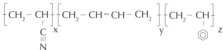
Akrylnitril
